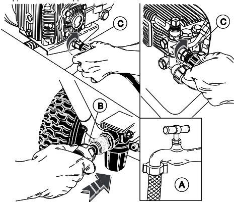
Подключение воды.
