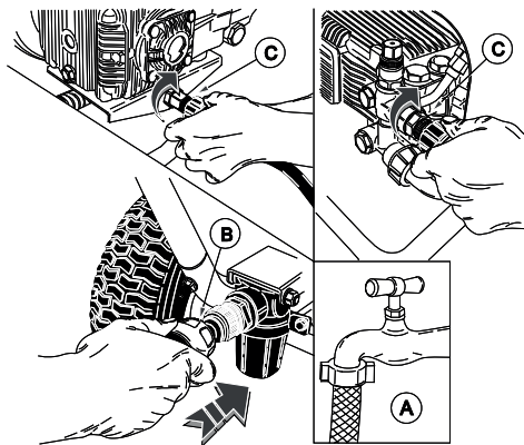
Wasseranschluß
