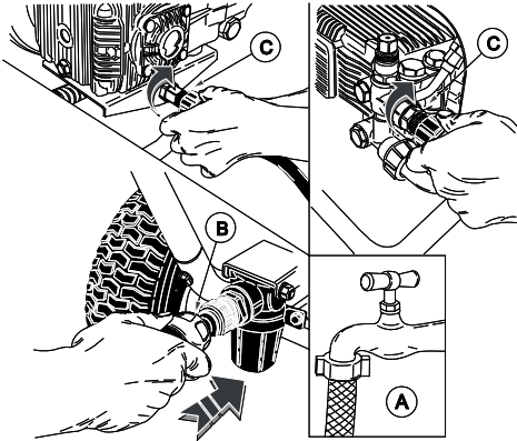
Conexión hídrica.
