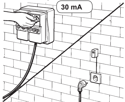
Branchement électrique.
