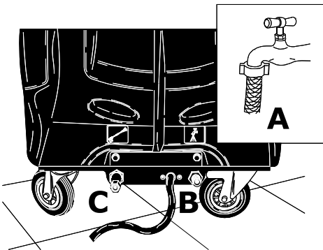
Подключение воды.
