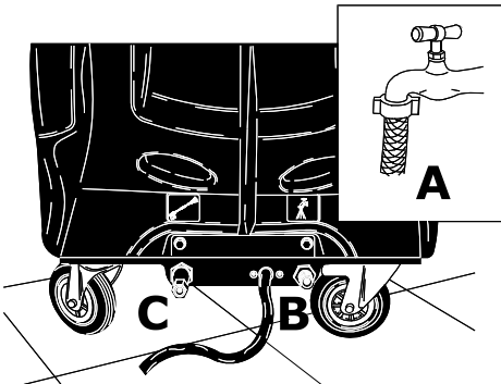
Collegamento idrico.
