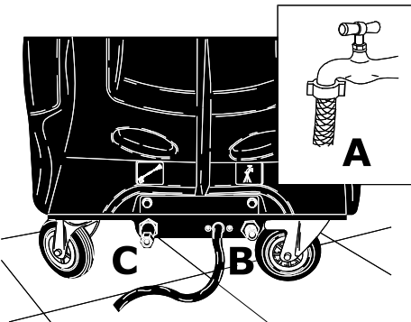
Conexión hídrica.
