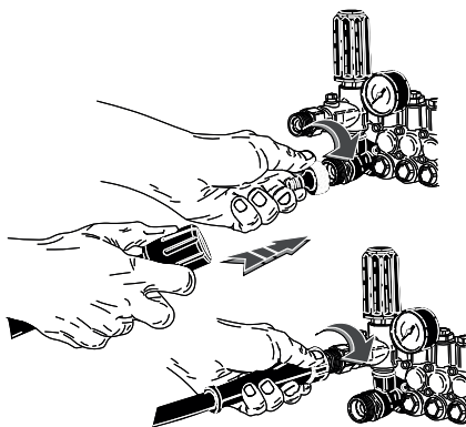
Подключение воды.
