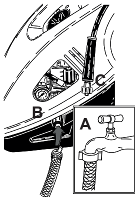
Collegamento idrico.
