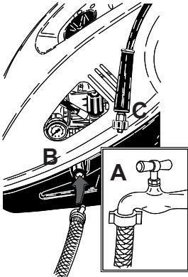
Wateraansluiting.
