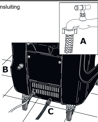
Wateraansluiting
