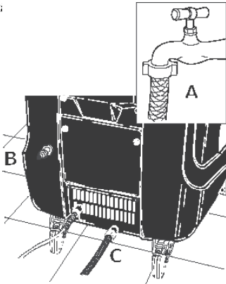
Vesiliitäntä:
