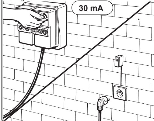
Collegamento elettrico.
